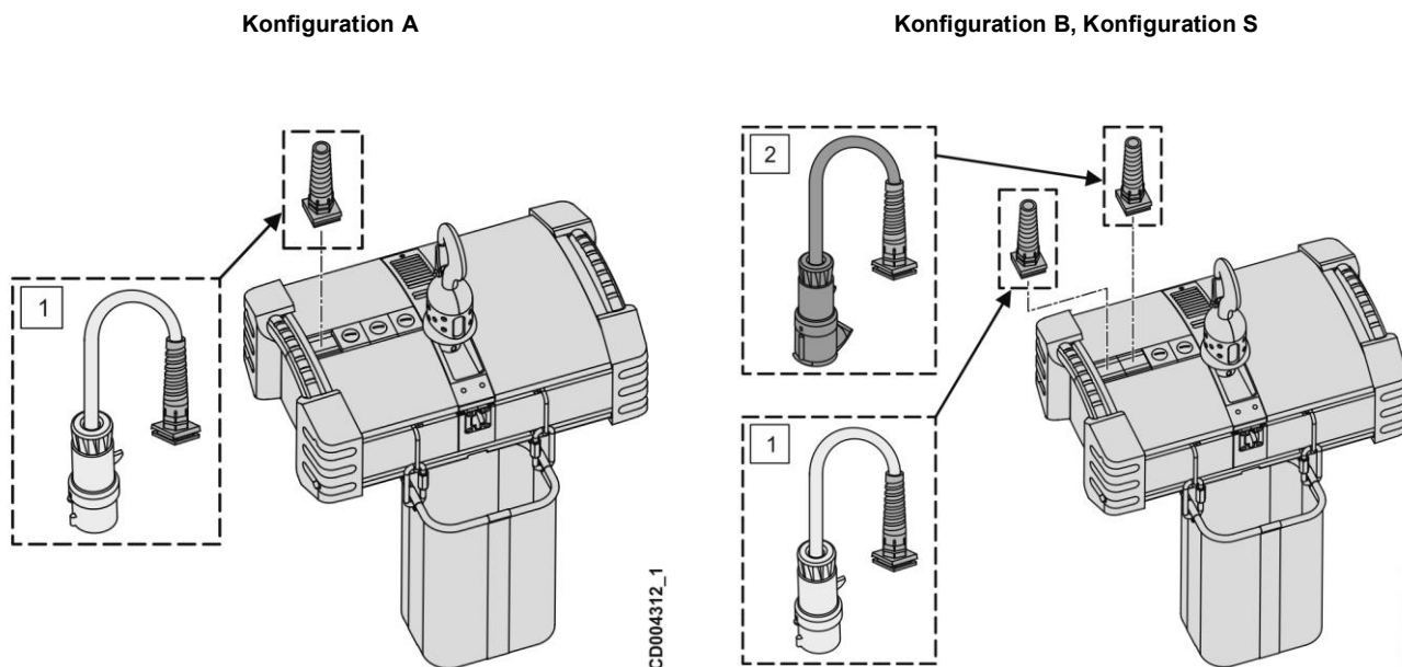
Figure 3. Beispiel für Kabeleingänge für Hubwerks-Stromversorgung und -Steuerung
